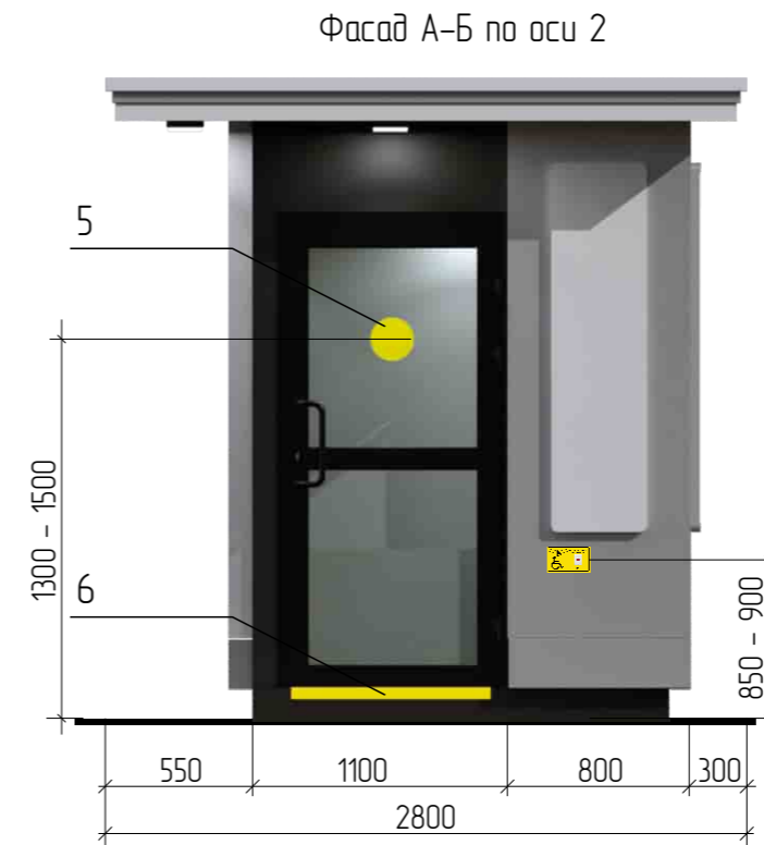
Общие виды павильона
