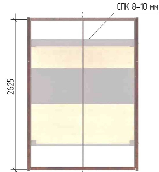
Торговая палатка 1.8x1,8x2.3 м (холодного типа)
