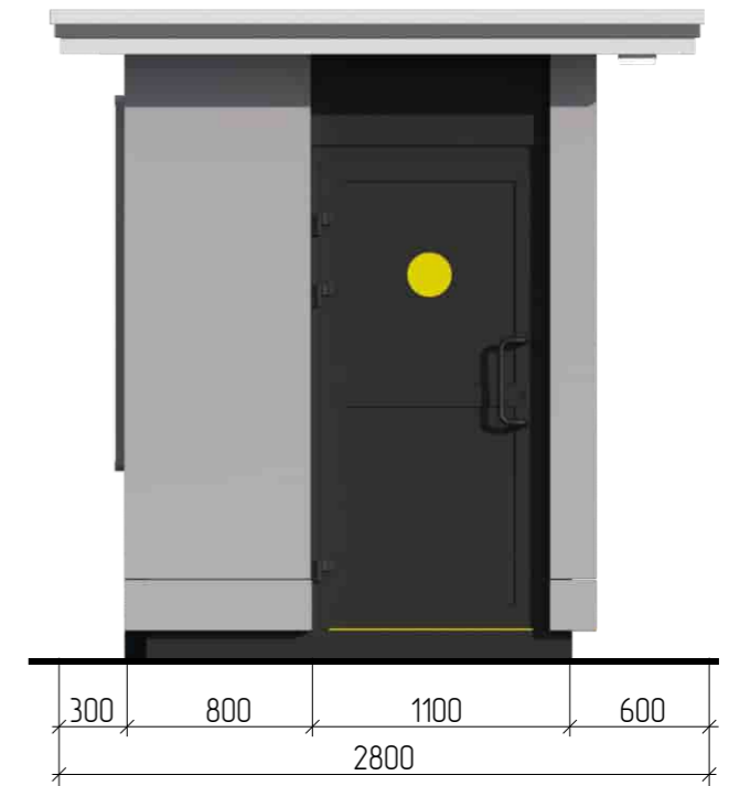
Фасад Б-А по оси 1
