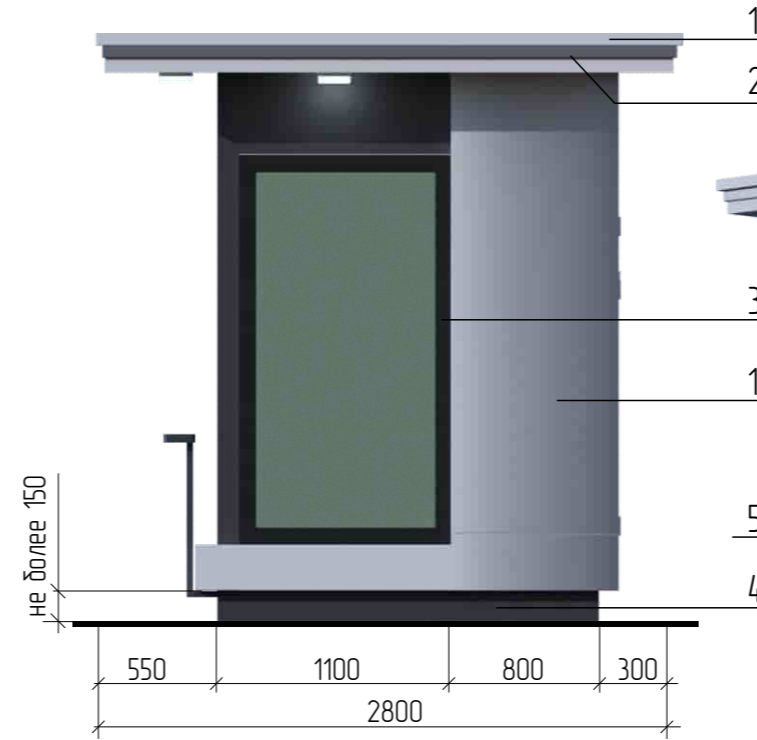
Фасад А-Б по оси 2
