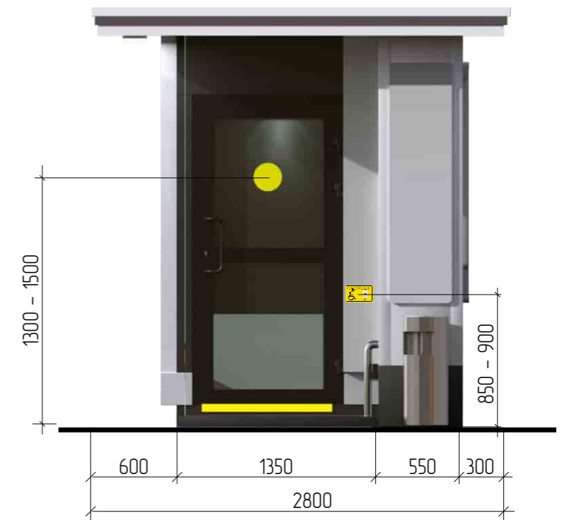
Фасад А-Б по оси 2
